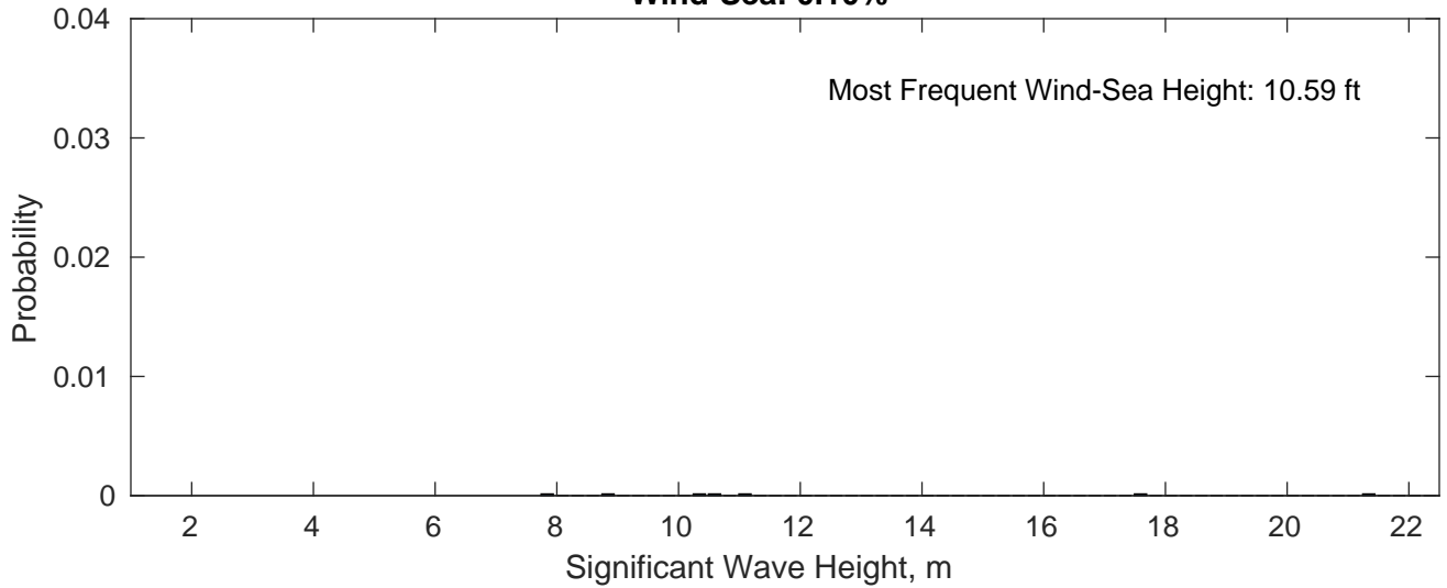
Wind-Sea: 0.10%
