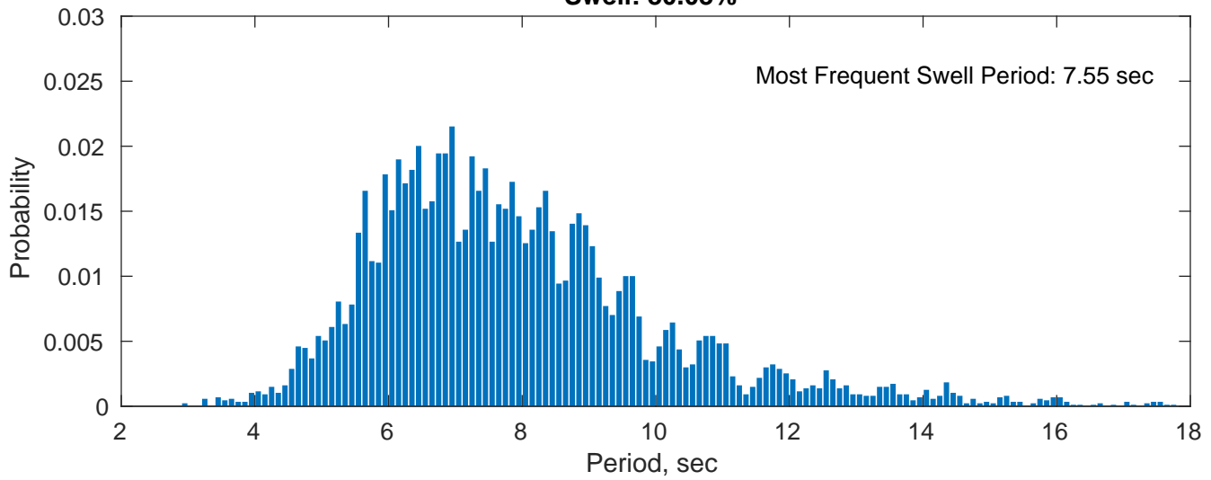
Swell: 80.03%
