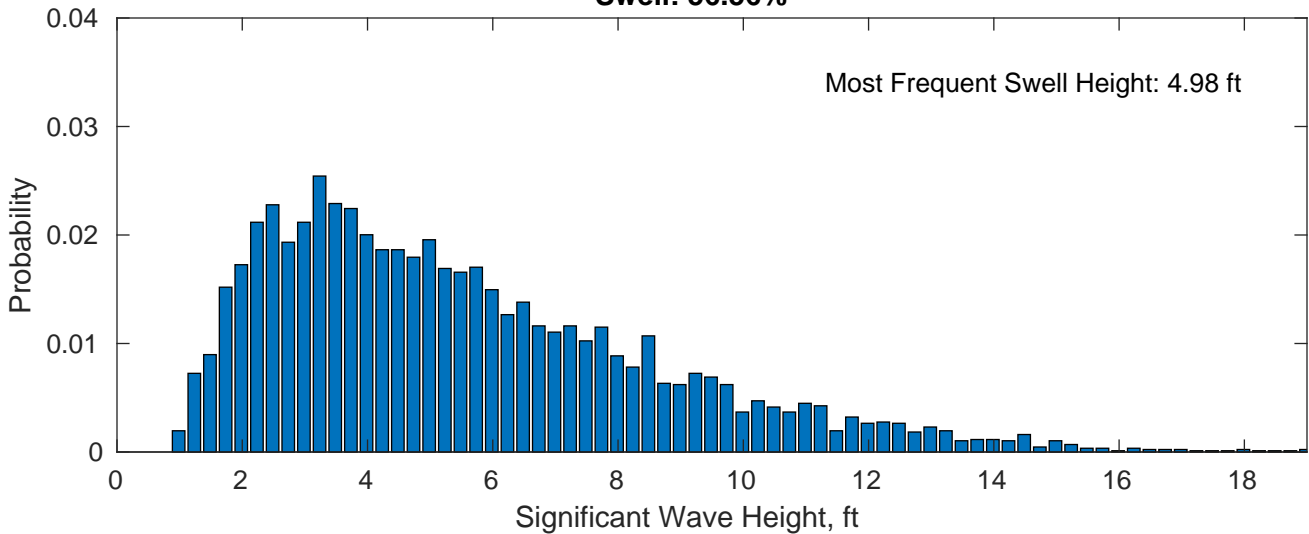
Swell: 56.56%
