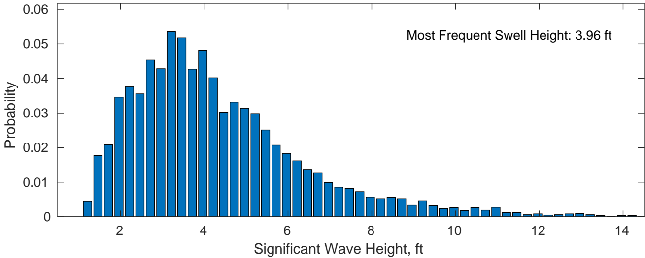
Swell: 79.87%
