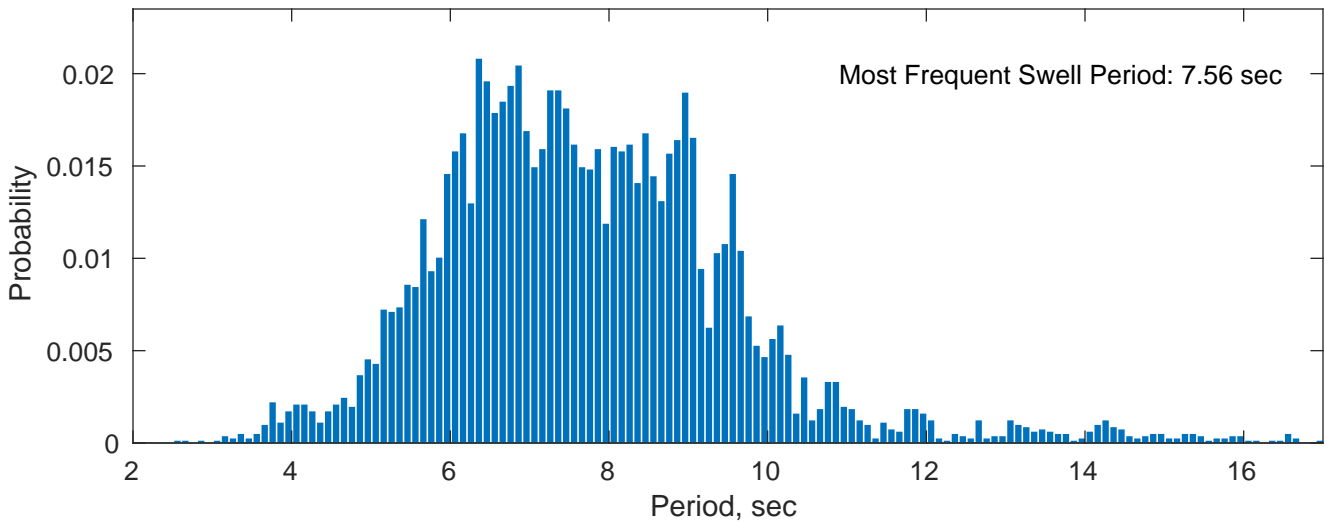
Swell: 78.23%
