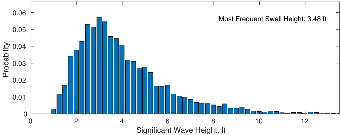
Swell: 79.07%
