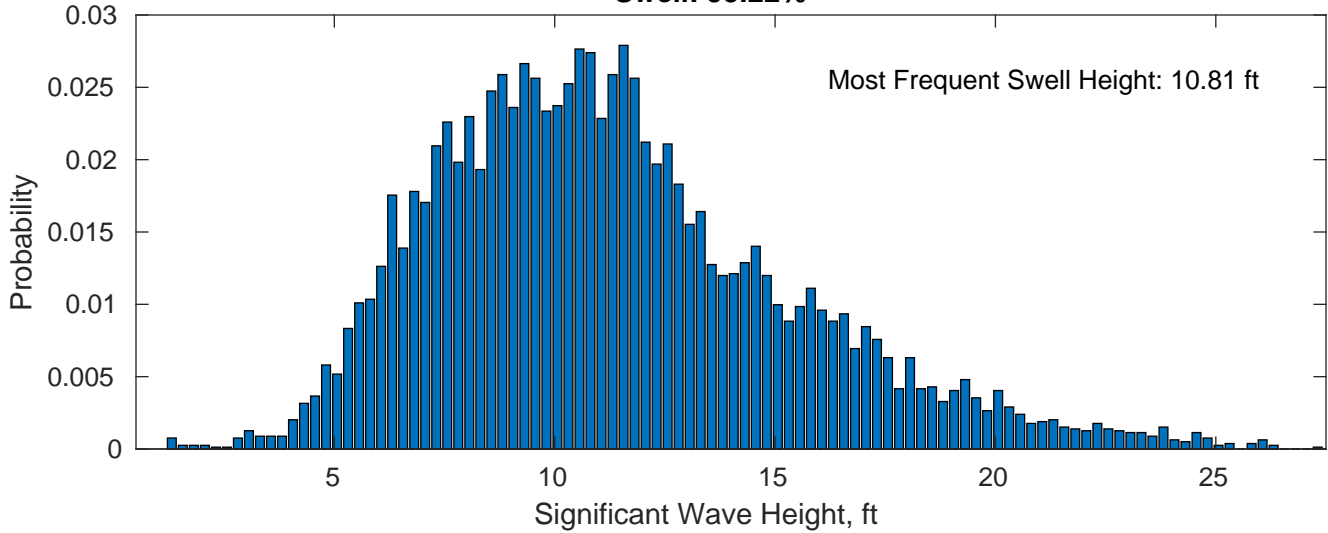
Swell: 95.22%
