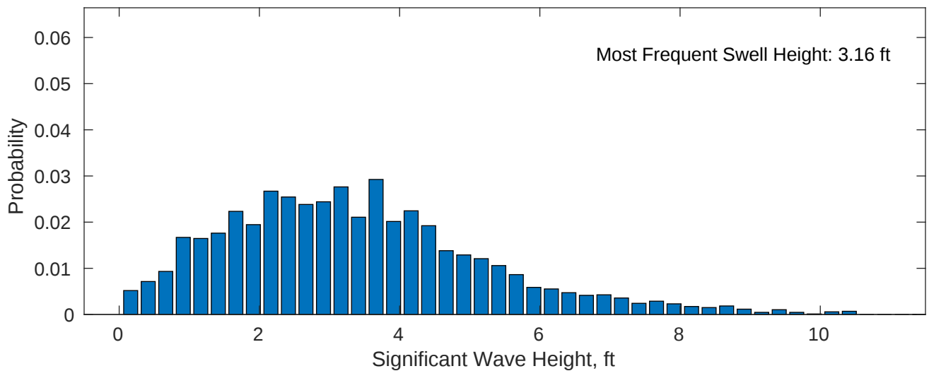
Swell: 45.77%
