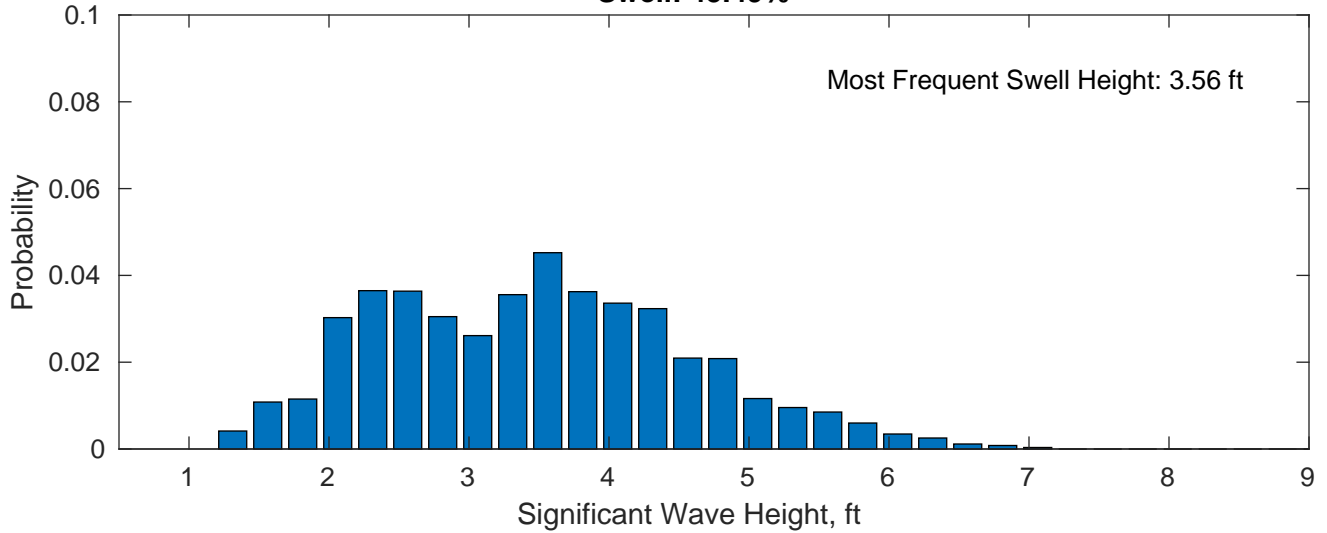
Swell: 45.49%
