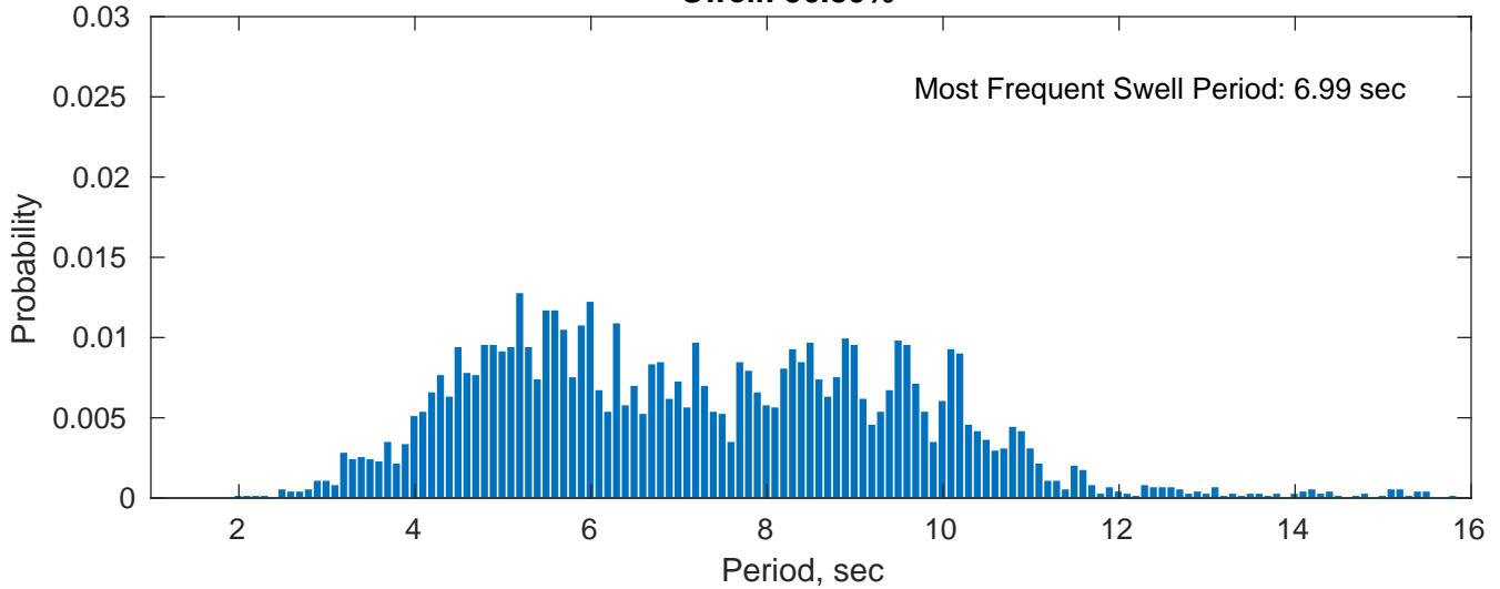
Swell: 56.80%
