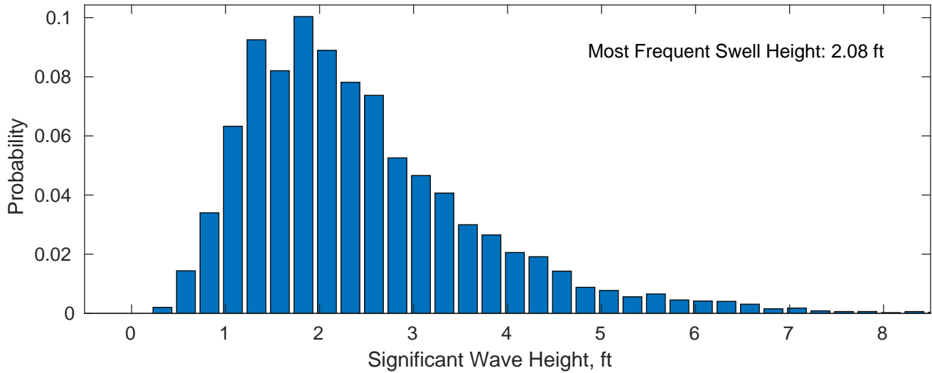
Swell: 93.41%
