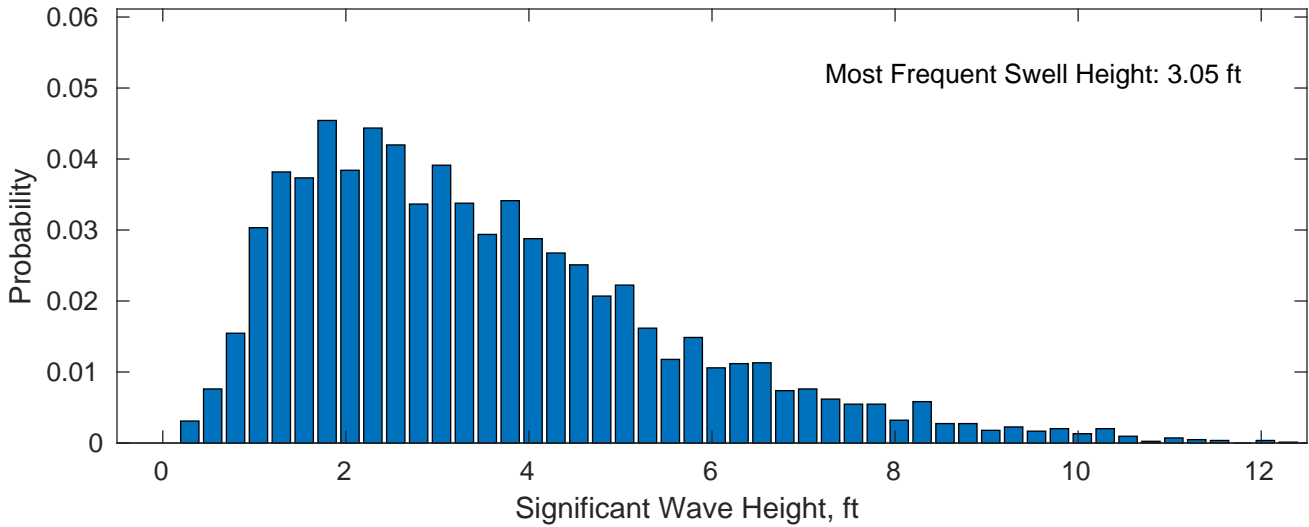
Swell: 73.33%
