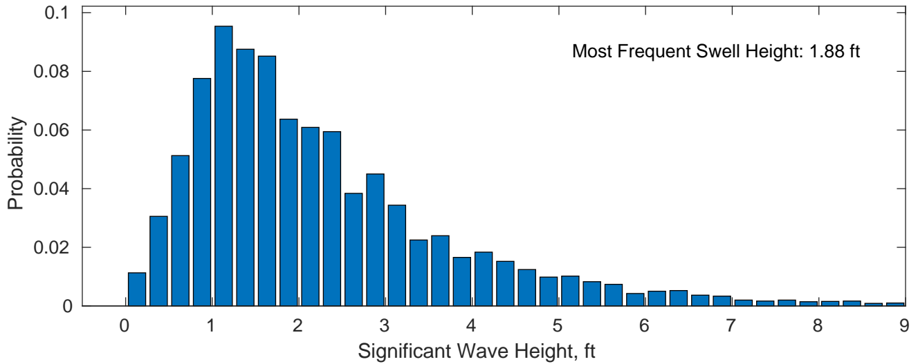
Swell: 92.21%
