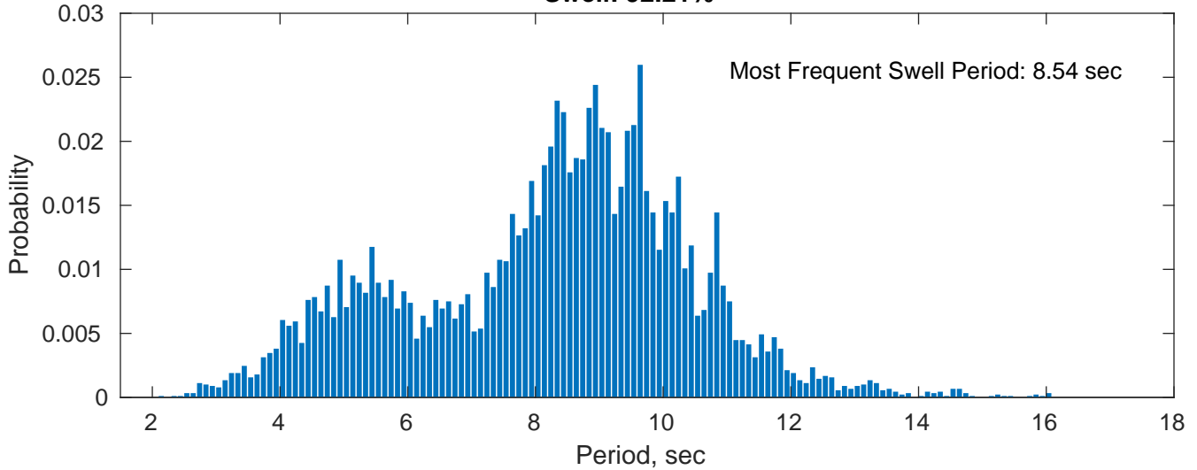
Swell: 92.21%
