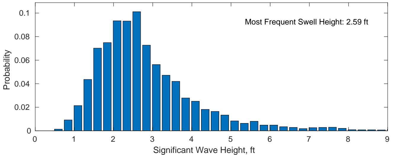
Swell: 88.63%
