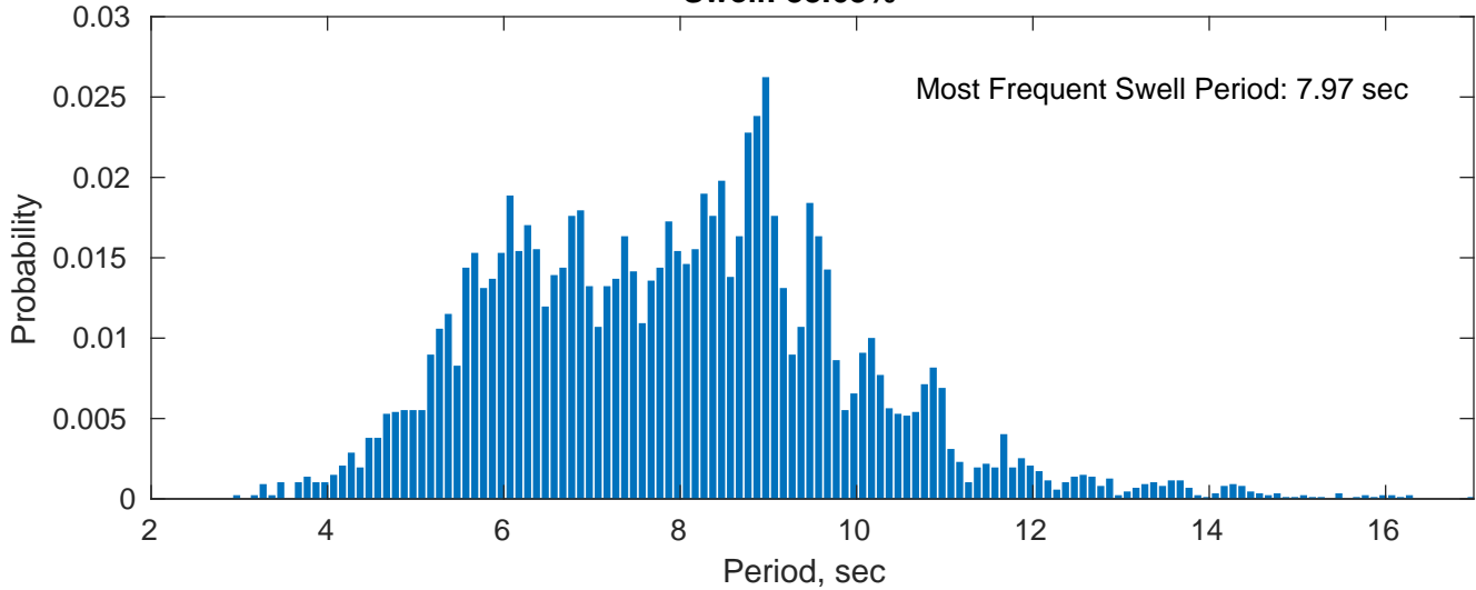
Swell: 88.63%
