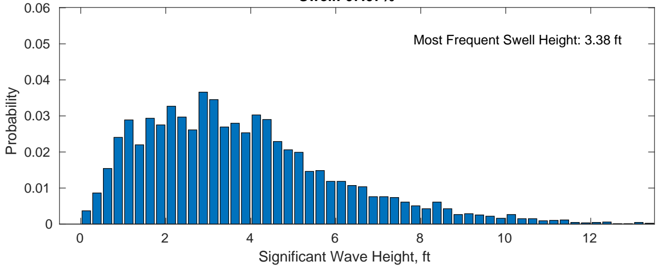
Swell: 67.07%
